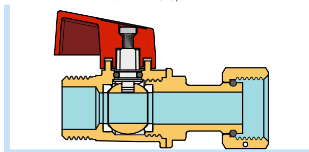
2941 - DETTAGLIO / DETAIL
