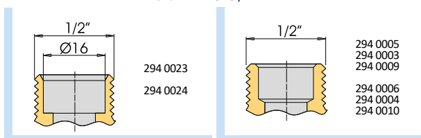
2946 - DETTAGLIO / DETAIL
